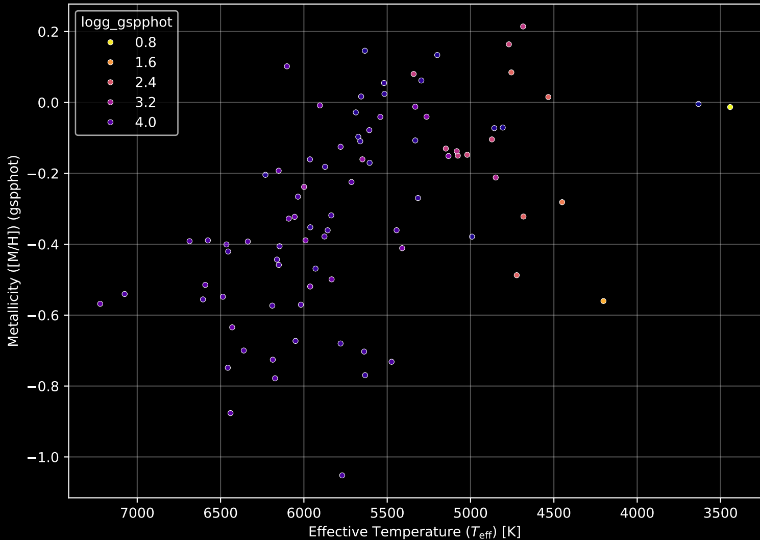
GALAH DR4 Field: [7176] Stellar Population Parameters (n= 87)
