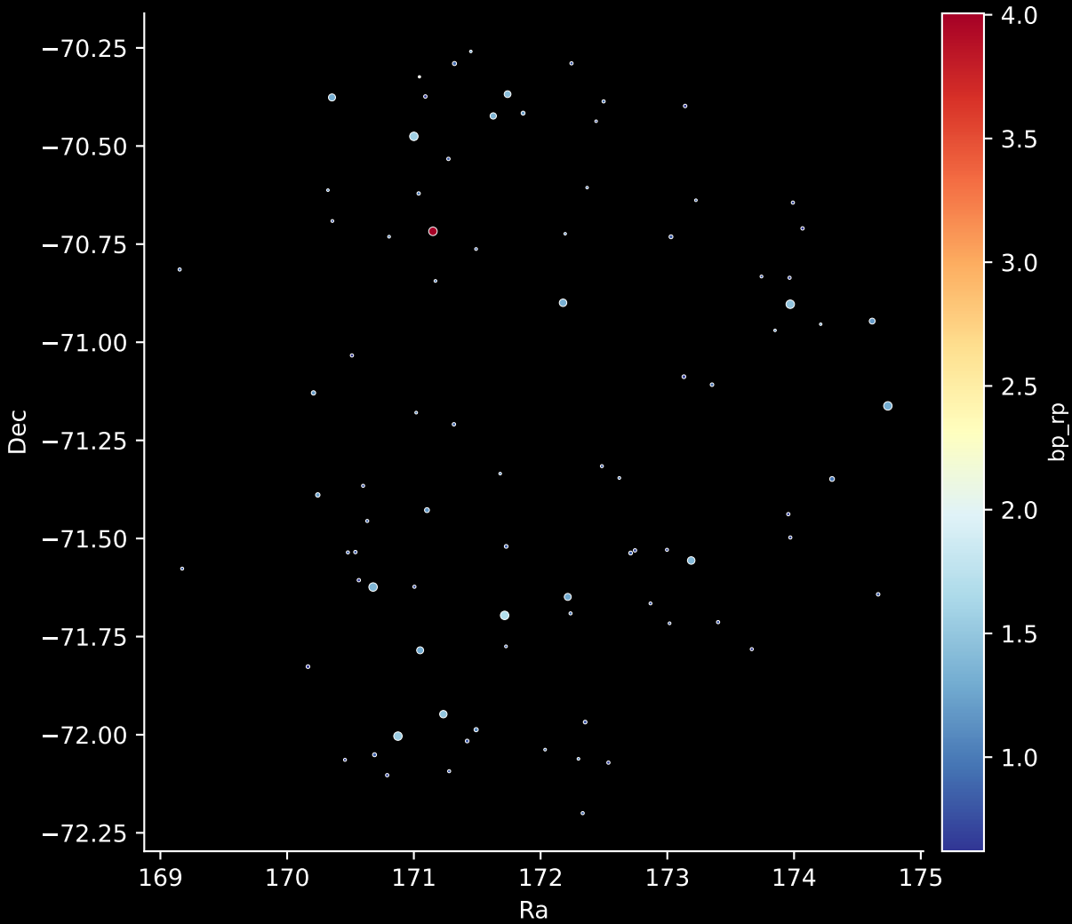
GALAH DR4 Field: [7176] Stars: 87
